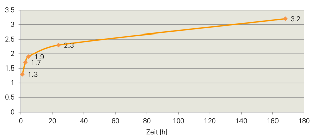
Kraftaufbau [N/mm 2 ]
